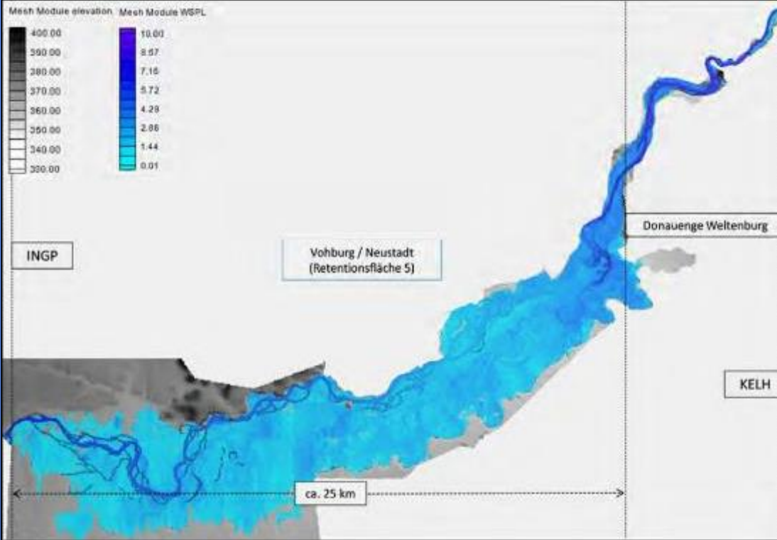
Abbildung IV - 21: Retentionsflächen an der historischen Donau zwischen Ingolstadt (INGP) und Kelheim (KELH).
