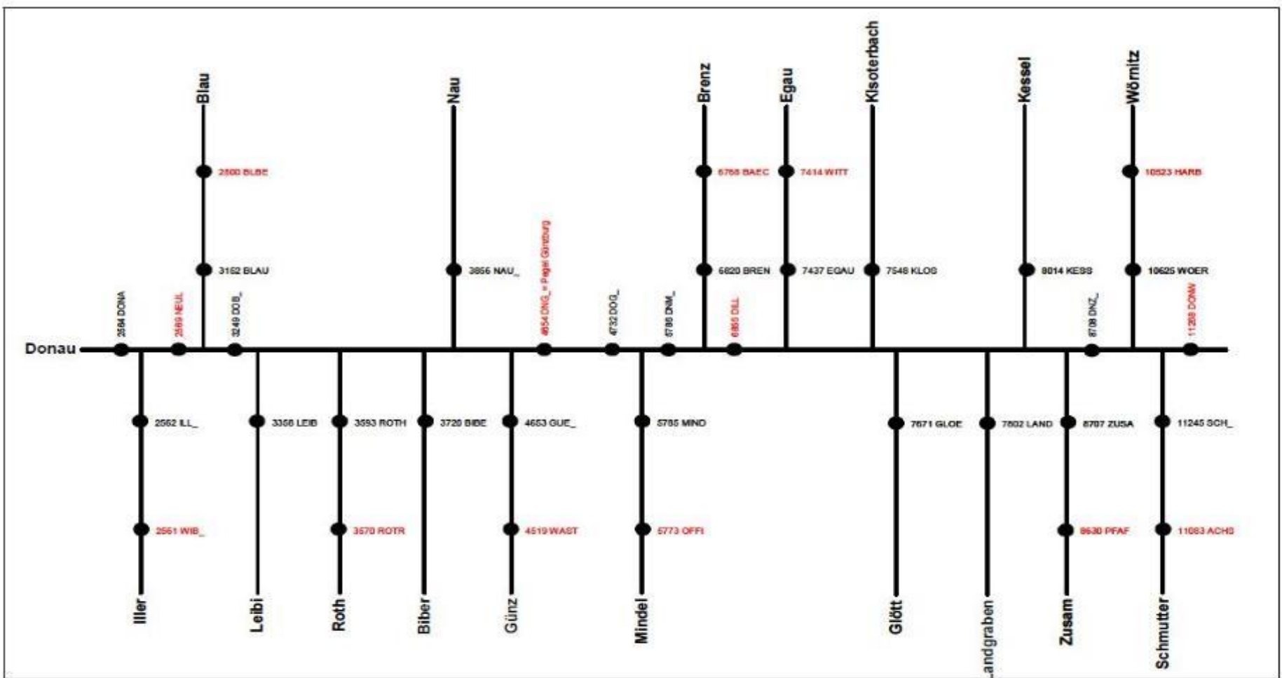
Abbildung 1: Gewässernetz und Ausgabeknoten
