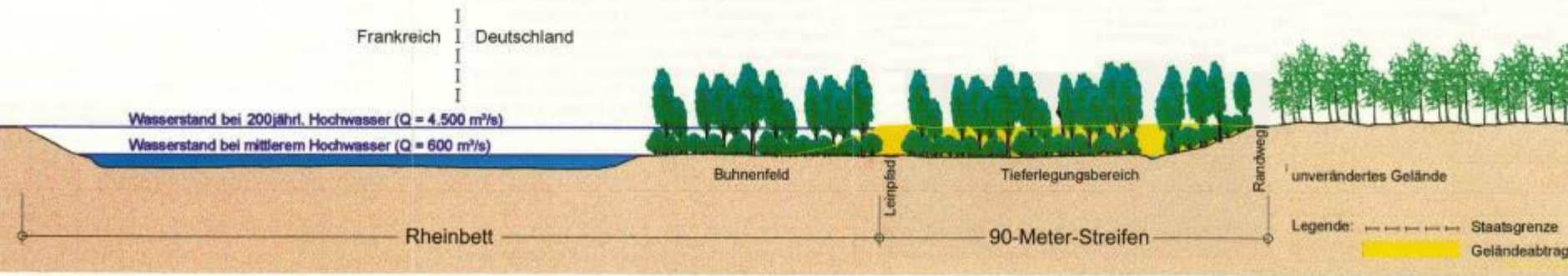
Querschnitt durch den Rhein mit geplanter Tieferlegung des sogenannten 90-Meter-Streifens
